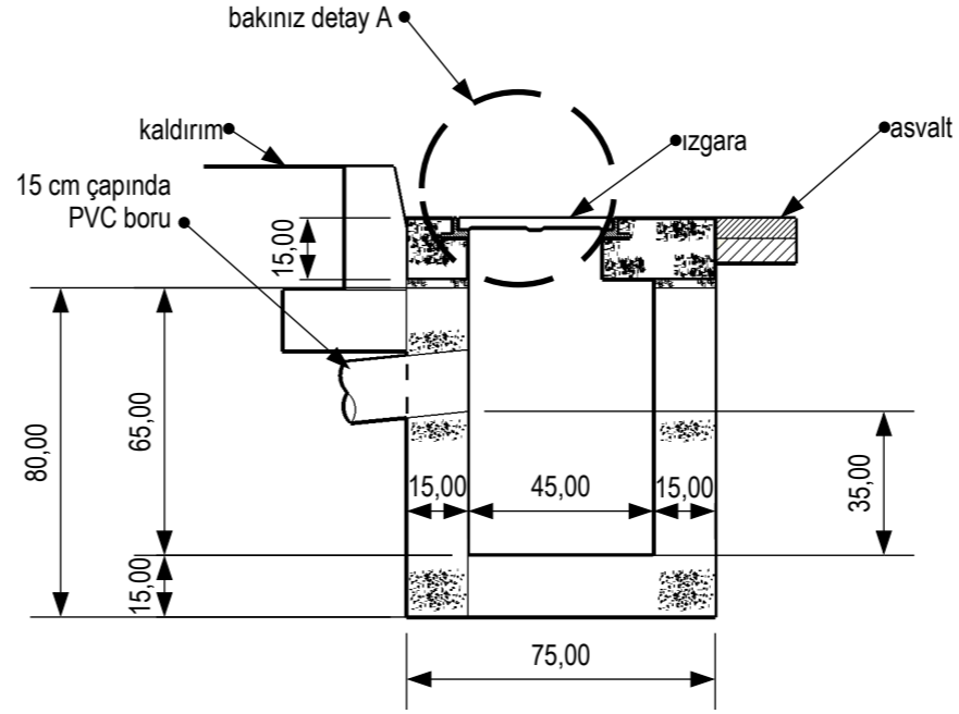
KESİT B - B
