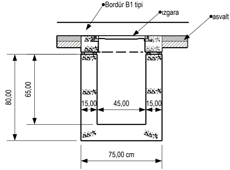
KESİT A - A
