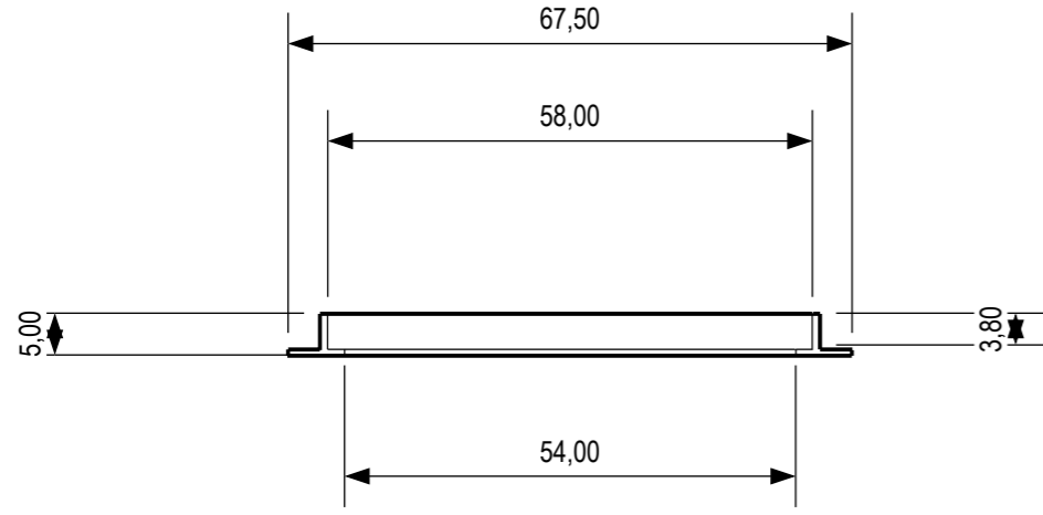
KESİT A - A
