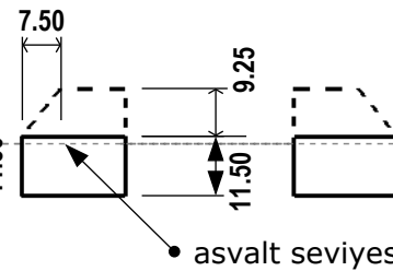
Yan Görünüş
